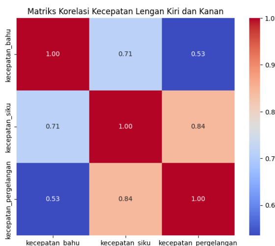
Gambar 11. Grafik korelasi antara lengan kiri dan kanan.
